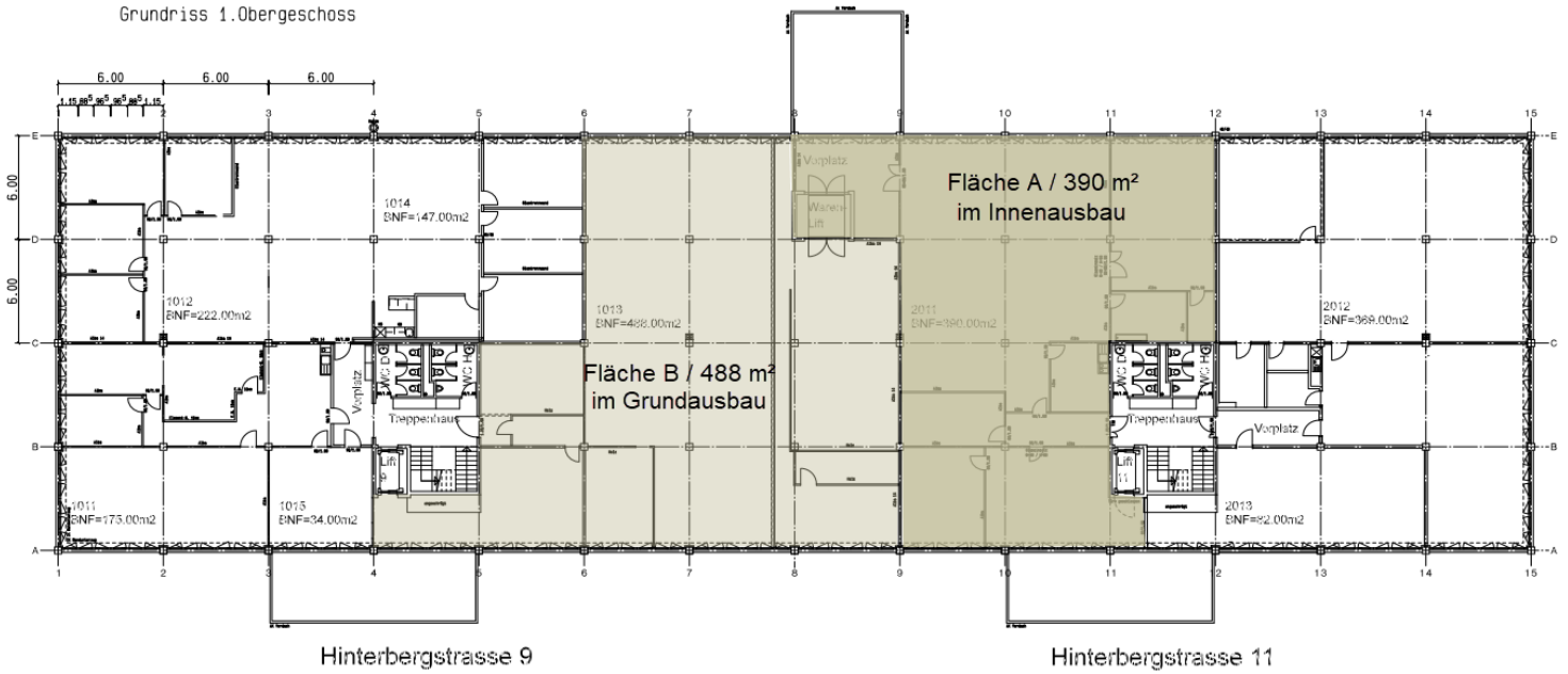
Grundriss 1.Obergeschoss
